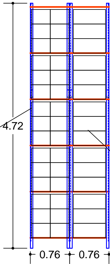
ELEVACION LATERAL
